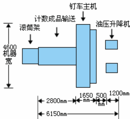
平面图
